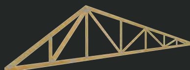
Wiązar asymetryczny
